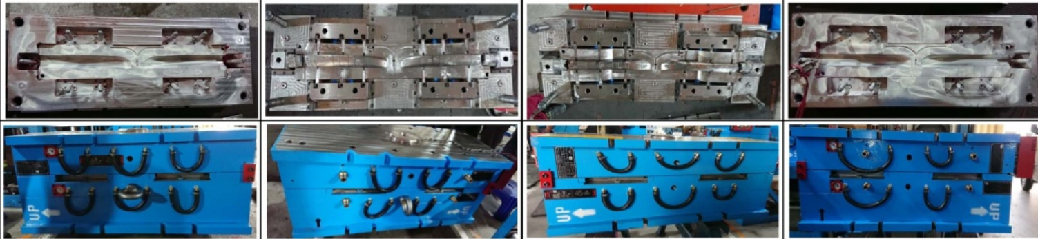
NU行李架前基座注塑模具(左/右)
